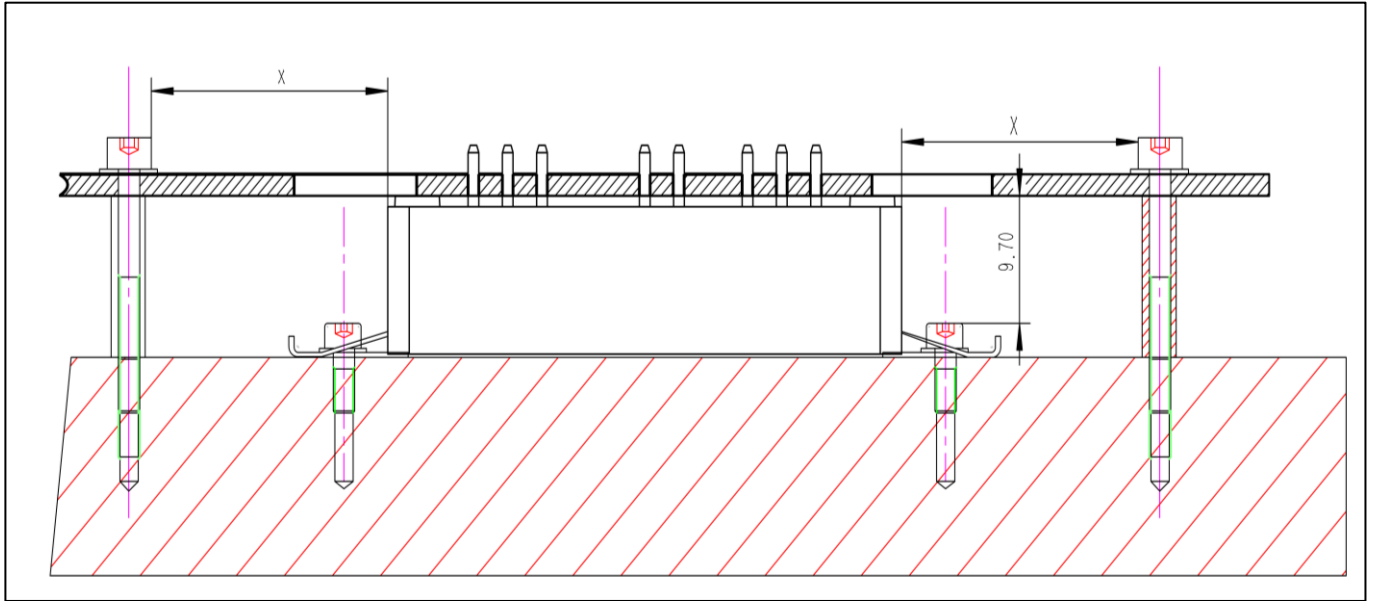
图7 PCB的固定
