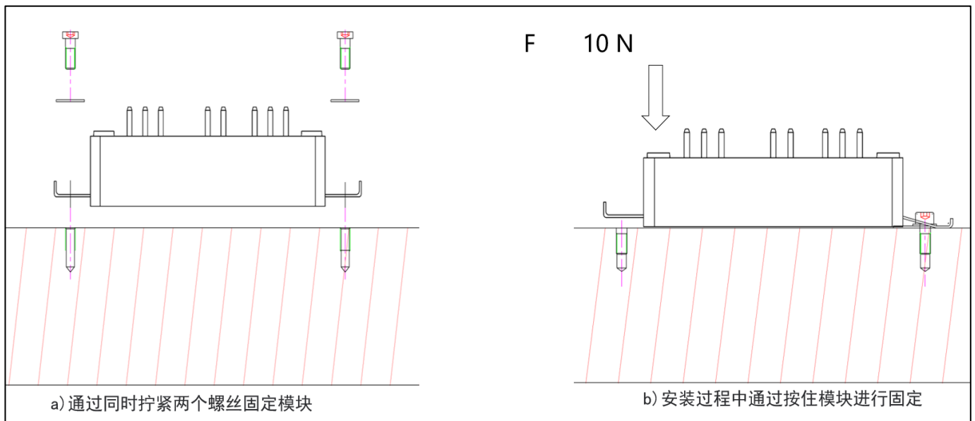
图6 将模块固定在散热器上
