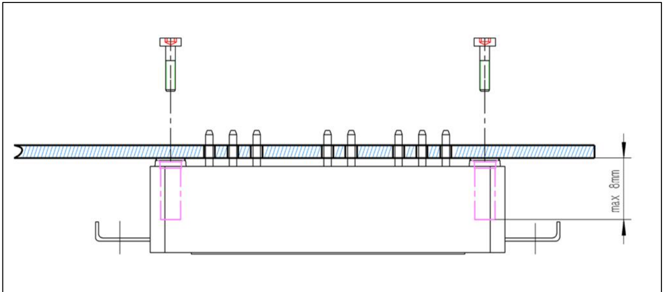
图4 使用螺栓进行PCB安装的示意图
