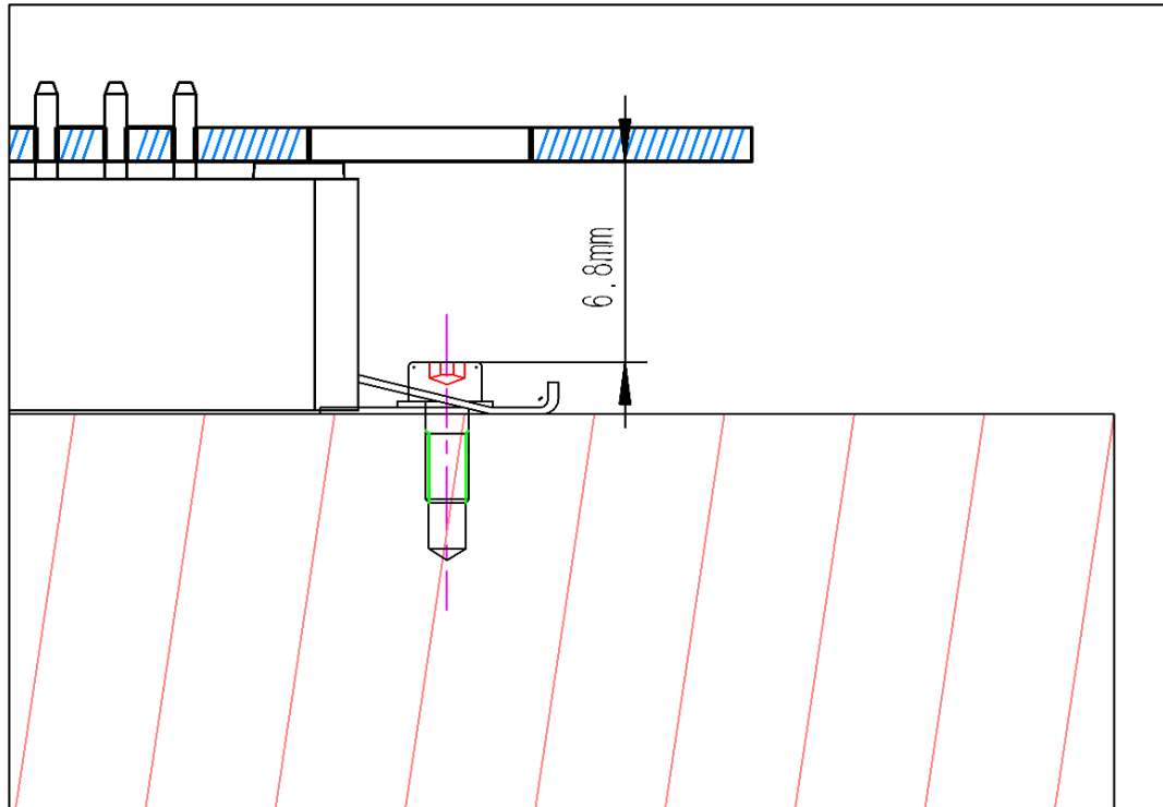
图9 螺丝夹和PCB之间的电气间隙
